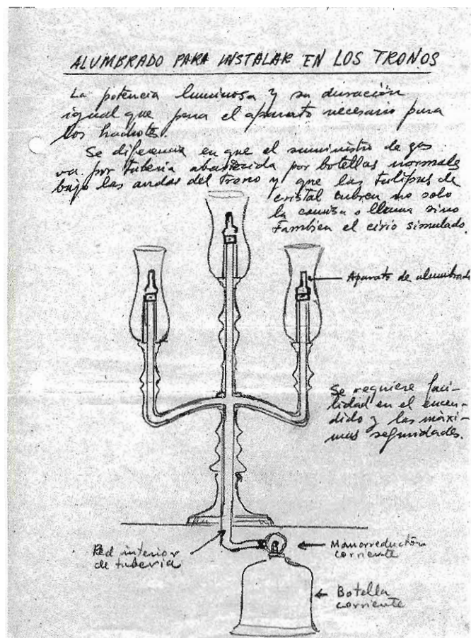
Boceto de alumbrado para instalar en tronos que se envió a distintas empresas de aparatos de gas. 14/02/1957.
