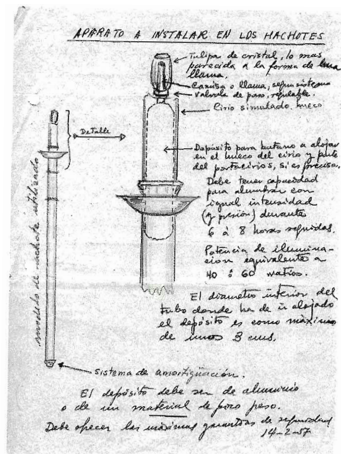
Boceto de alumbrado para instalar en los hachotes que se envió a distintas empresas de aparatos de gas. 14/02/1957.
