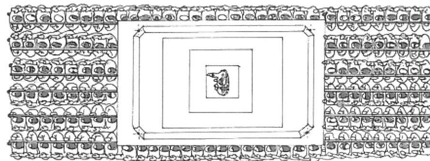
Distribución de los 134 portapasos en función del nuevo número de varas y del reparto de cargas.
