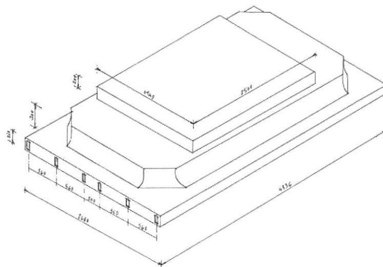
Plano isométrico de la plataforma del trono, con la nueva disposición de los tres cajones.
