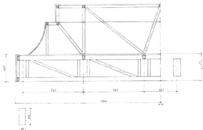
Diseño de la celosía empleada para la estructura del nuevo trono.
